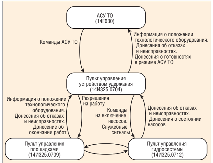
Рис. 4. Функциональные связи оборудования системы управления
