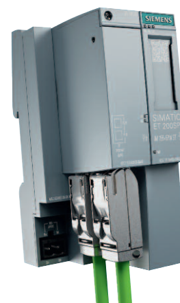
Рис. 2. Головной интерфейсный модуль с сетевым адаптером 2×RJ-45
