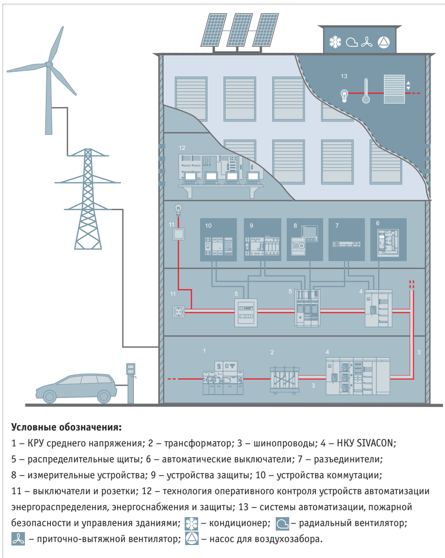
Рис. 5. Комплексная система управления зданием, включающая интегрированные решения по распределению электроэнергии, автоматизации здания и пожарной безопасности
