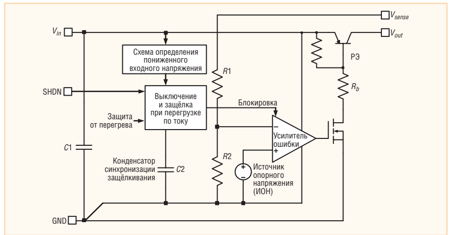
Рис. 2. Упрощённая схема ЛСН серии IRUN330118AК/AP без функции регулировки выходного напряжения (в стабилизаторе с регулировкой выходного напряжения верхний резистор делителя отсутствует и к средней точке делителя напряжения подключается внешний резистор – вывод V_{sense} заменяется на вывод внешнего резистора ADJ)
