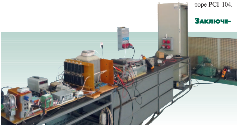
Рис. 7. Испытательный стенд преобразователя Momentum
