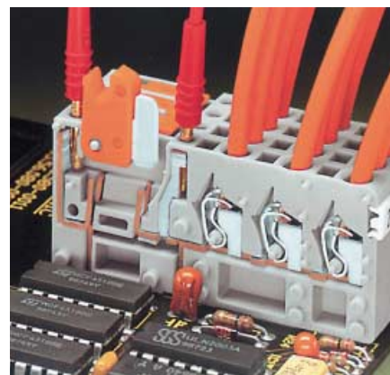
Рис. 6. Трёхполюсные клеммы для печатных плат на базе ССС серии 742
